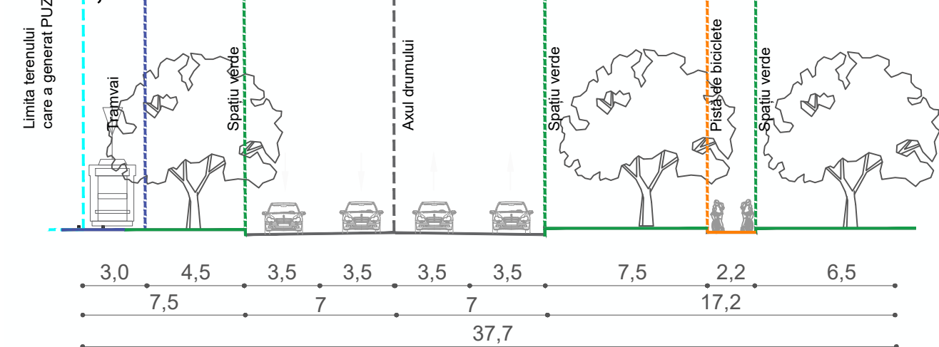
SECȚIUNE CĂLEA ZIMANDULUI A-A' sc. 1:250
